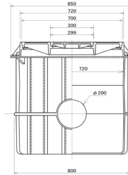
A-A断面 量水器ボックス配管部パッキン
