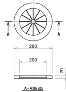
A-A断面 量水器ボックス配管部パッキン
