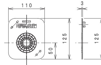
④ 土留板
