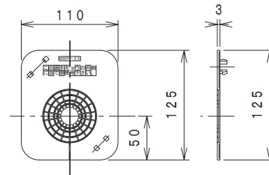
④ 土留板
