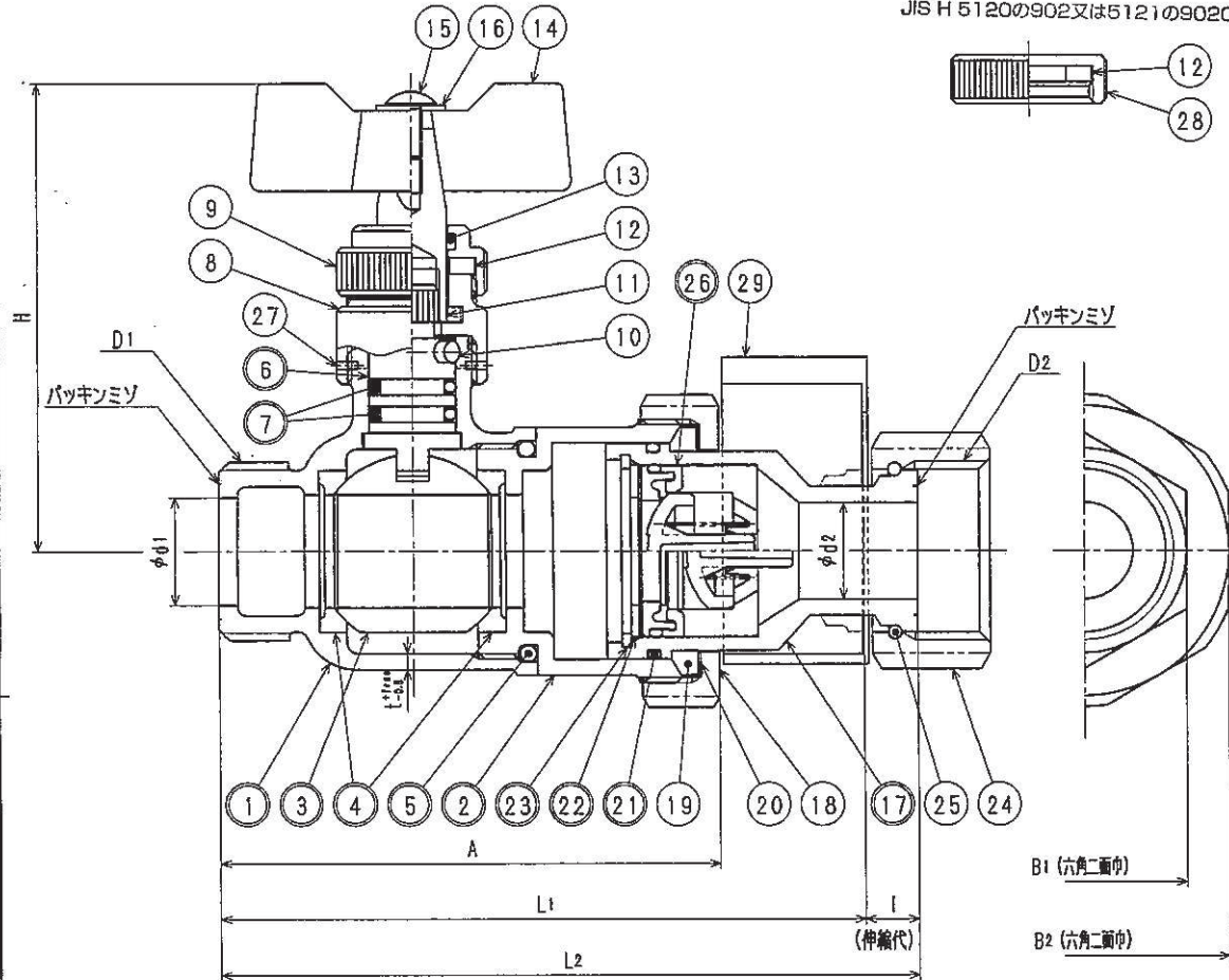
寸法表
